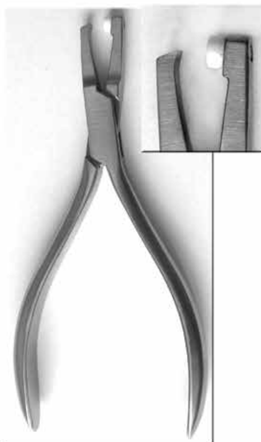
OD 1306 14 cm GYŰRŰ LEVEVŐ FOGÓ TEFLON BETÉTTTEL BAND-ABNEHME ZANGE MIT TEFLON EINZATZ BAND REMOVING PLIERS WITH TEFLON INSERT
